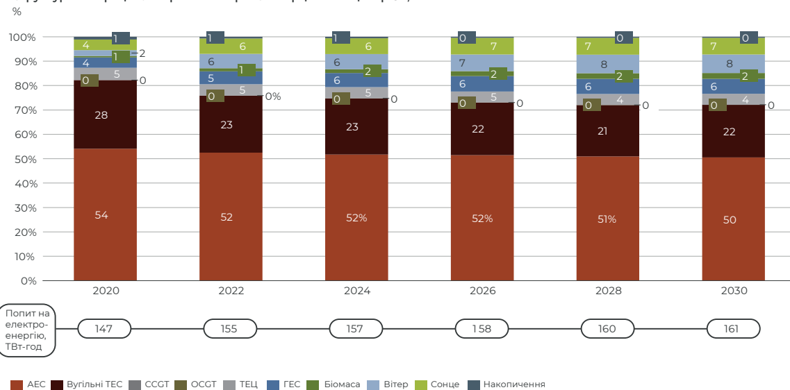
Структура генерації електричної енергії за інерційним сценарієм,
