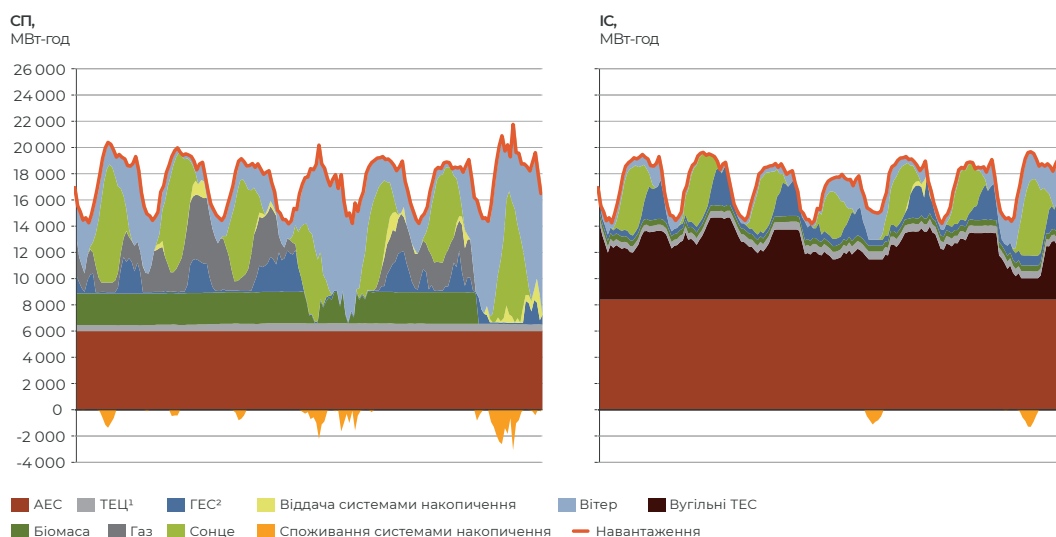
Профіль погодинної генерації електроенергії у період 20–27 червня 2030 року
