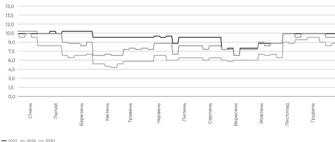
Погодинна генерація електроенергії атомними електростанціями за сценарієм переходу, ГВт-год
