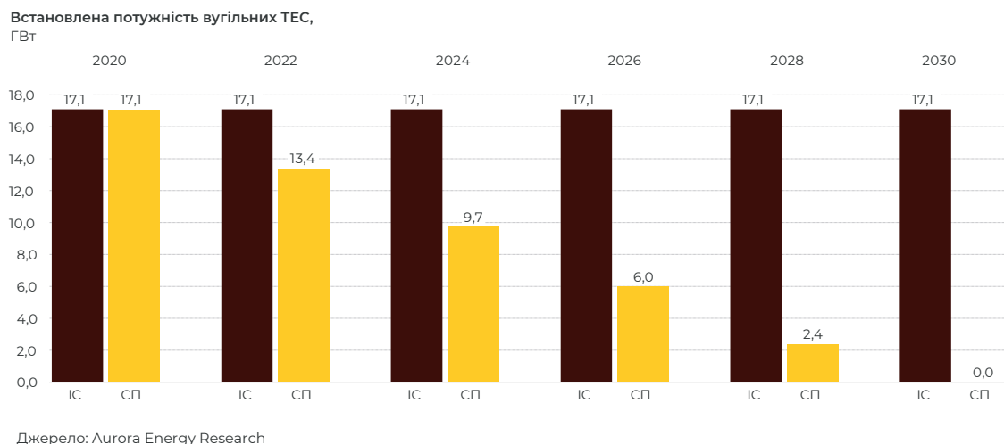
Рисунок 9. Встановлена потужність вугільної електроенергетики за IC та СП
