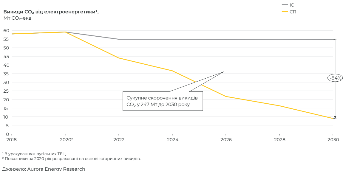
Рисунок 24. Викиди електроенергетичного сектору в період 2020–2030 років за двома сценаріями
