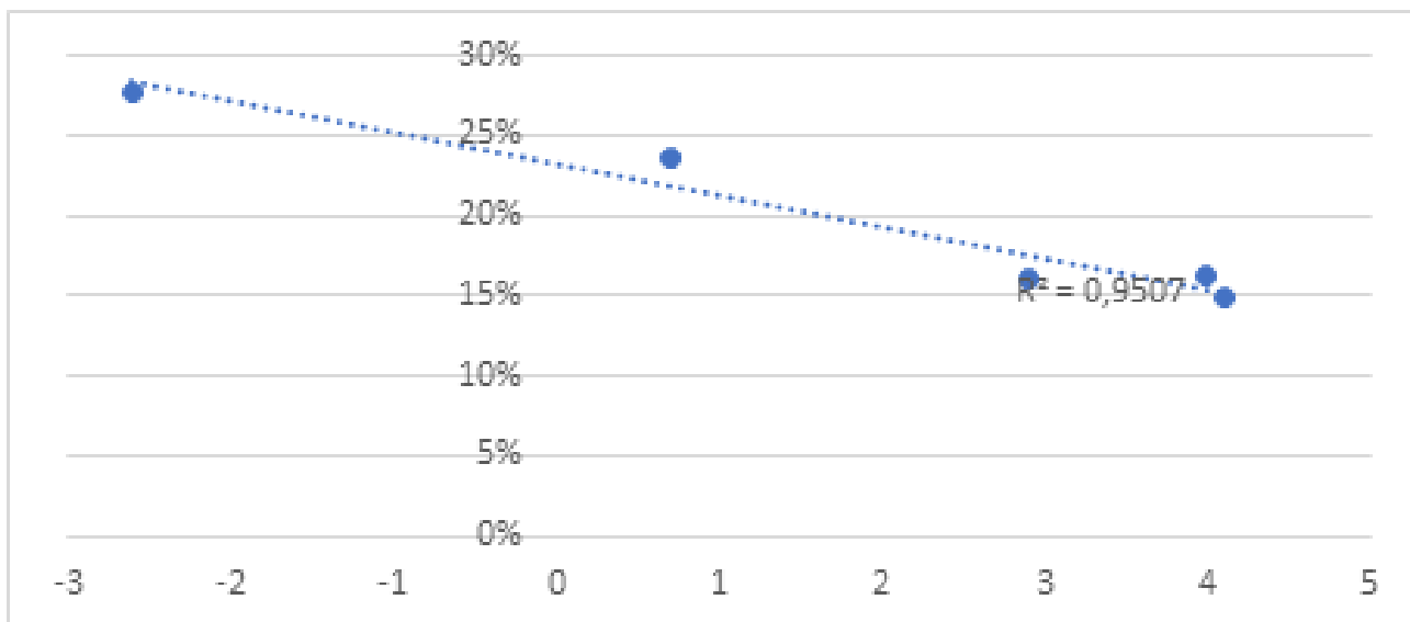
Рис. 3 Приклад ефективного регулювання, коли споживання має сильну кореляцію з зовнішньою температурою.
