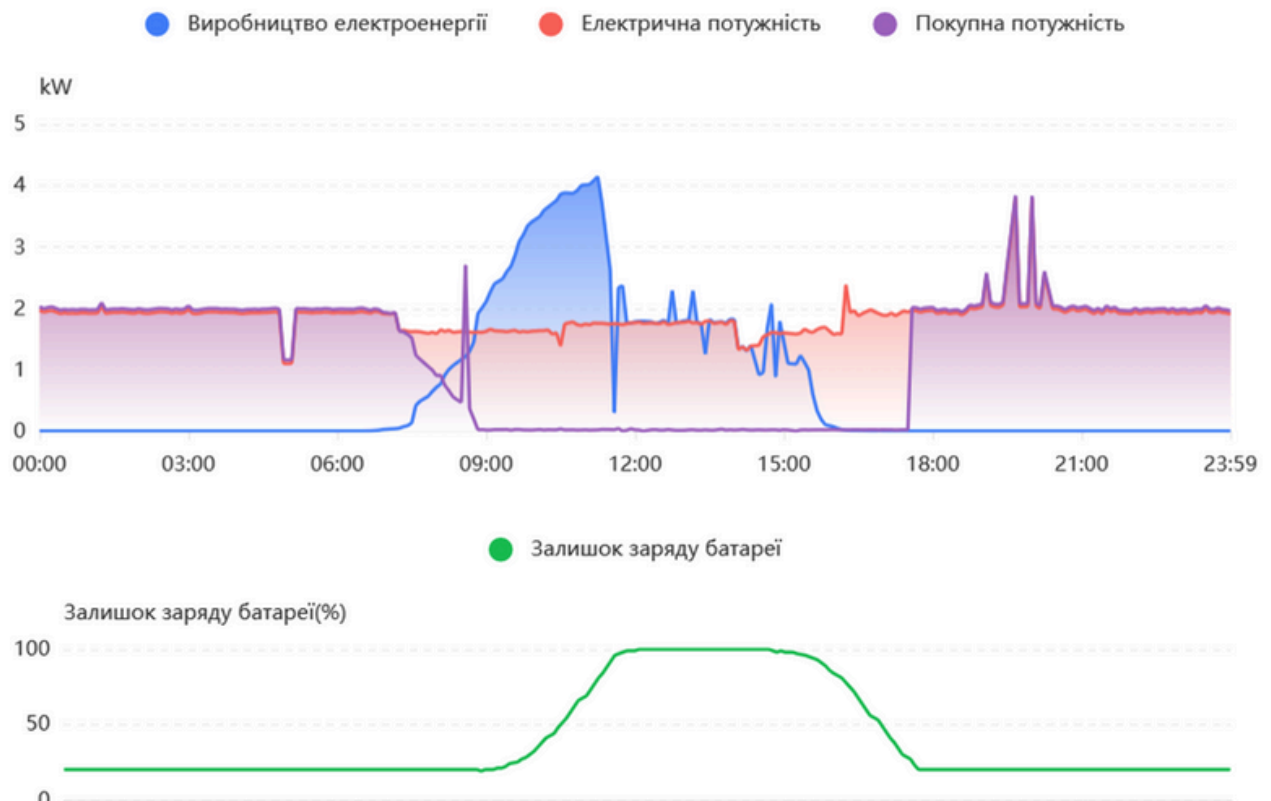
Рис. 9 Графік споживання електроенергії в «зимовому режимі»
