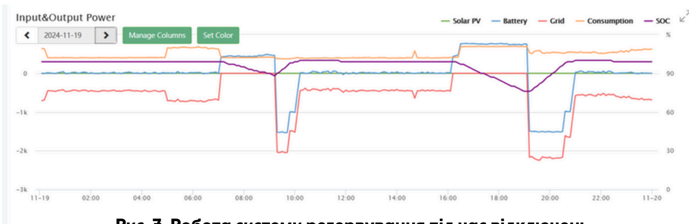
Рис. 7. Робота системи резервування під час відключень.
