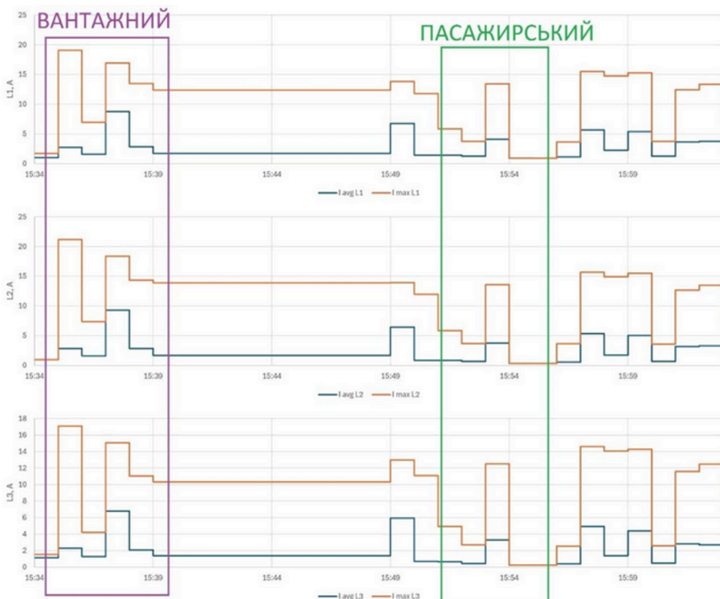
Рис. 1. Результати замірів пускових струмів під час роботи ліфтів (нерегульований привід)
