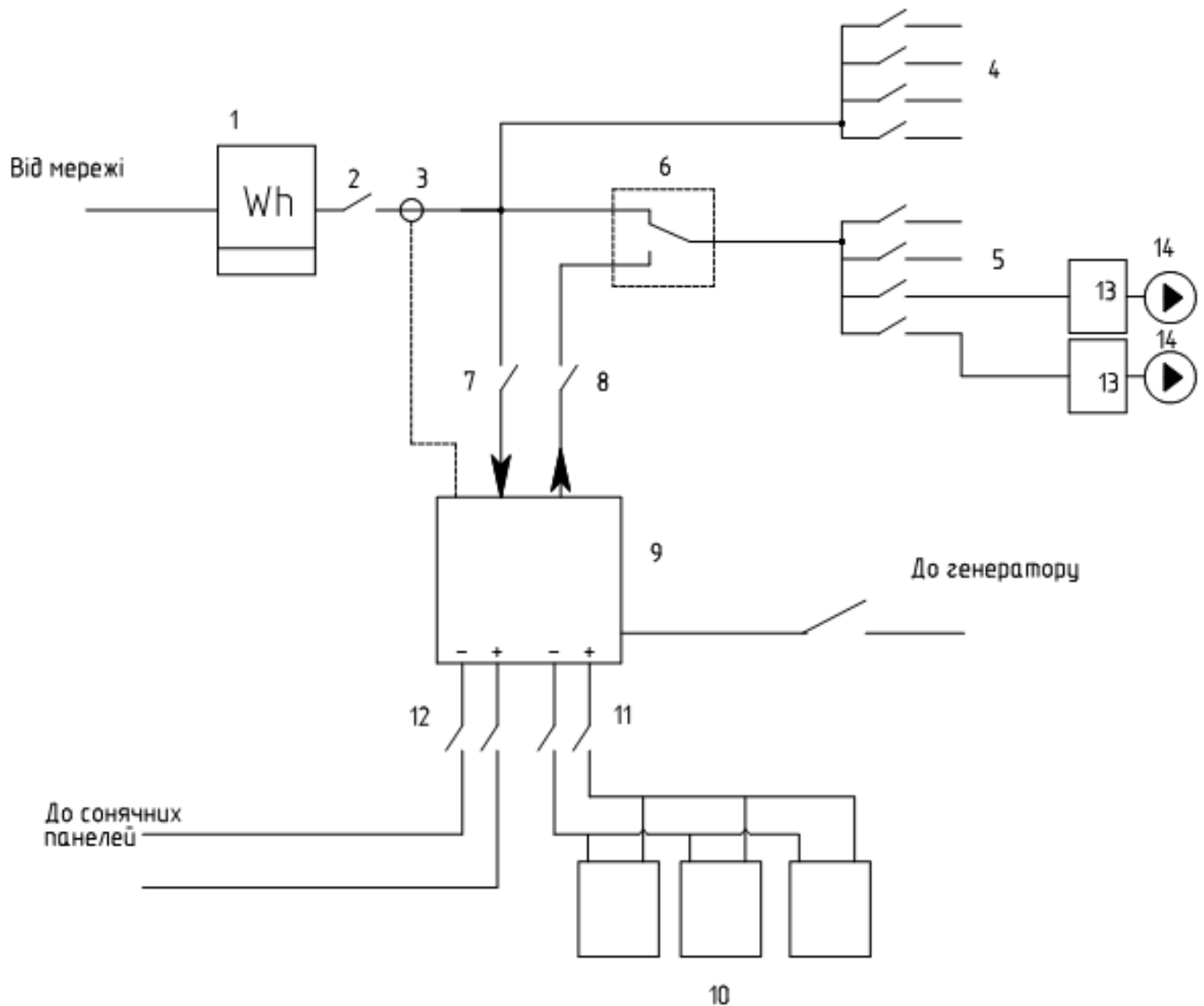
Рис. 2. Схема включення гібридного інвертора в схему живлення загальнобудинкових потреб з дооснащенням насосного обладнання частотними перетворювачами
