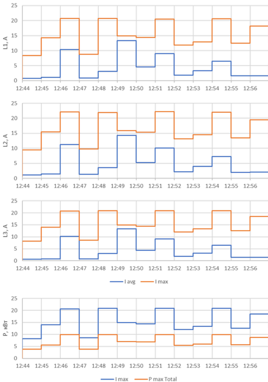
Рис. 4. Результати замірів пускових струмів під час роботи ліфту 400 кг з перетворювачами частоти
