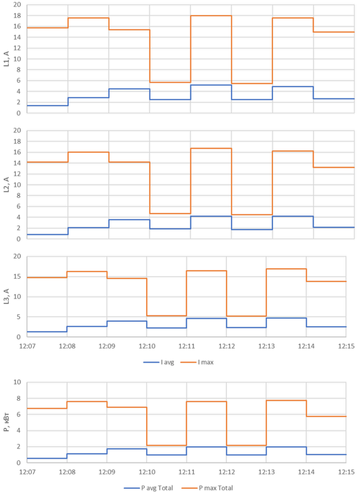
Рис. 3. Результати замірів пускових струмів під час роботи ліфту 400 кг з частотними регулювачами
