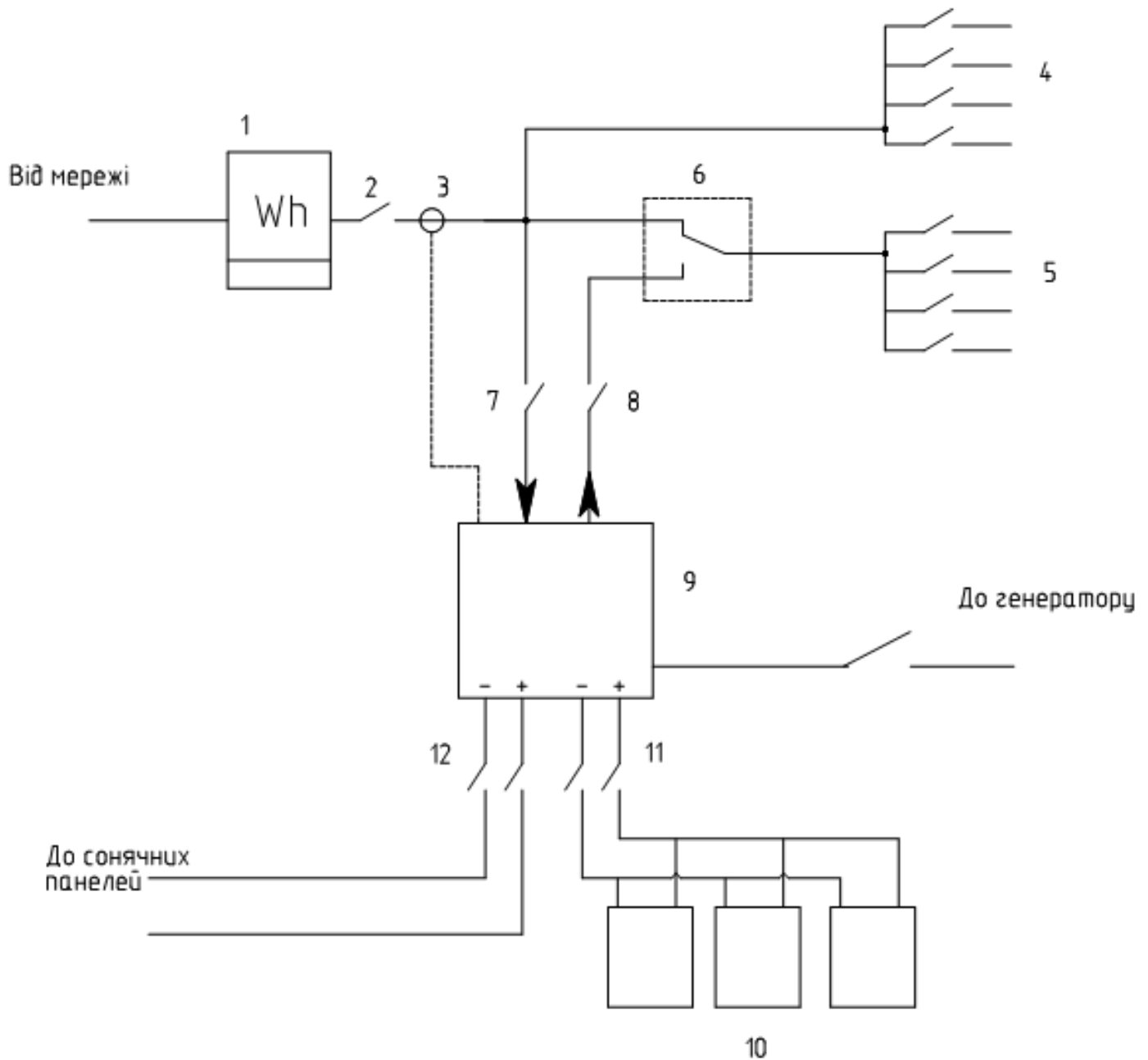
Рис. 1. Схема включення гібридного інвертора в схему живлення загальнобудинкових потреб
