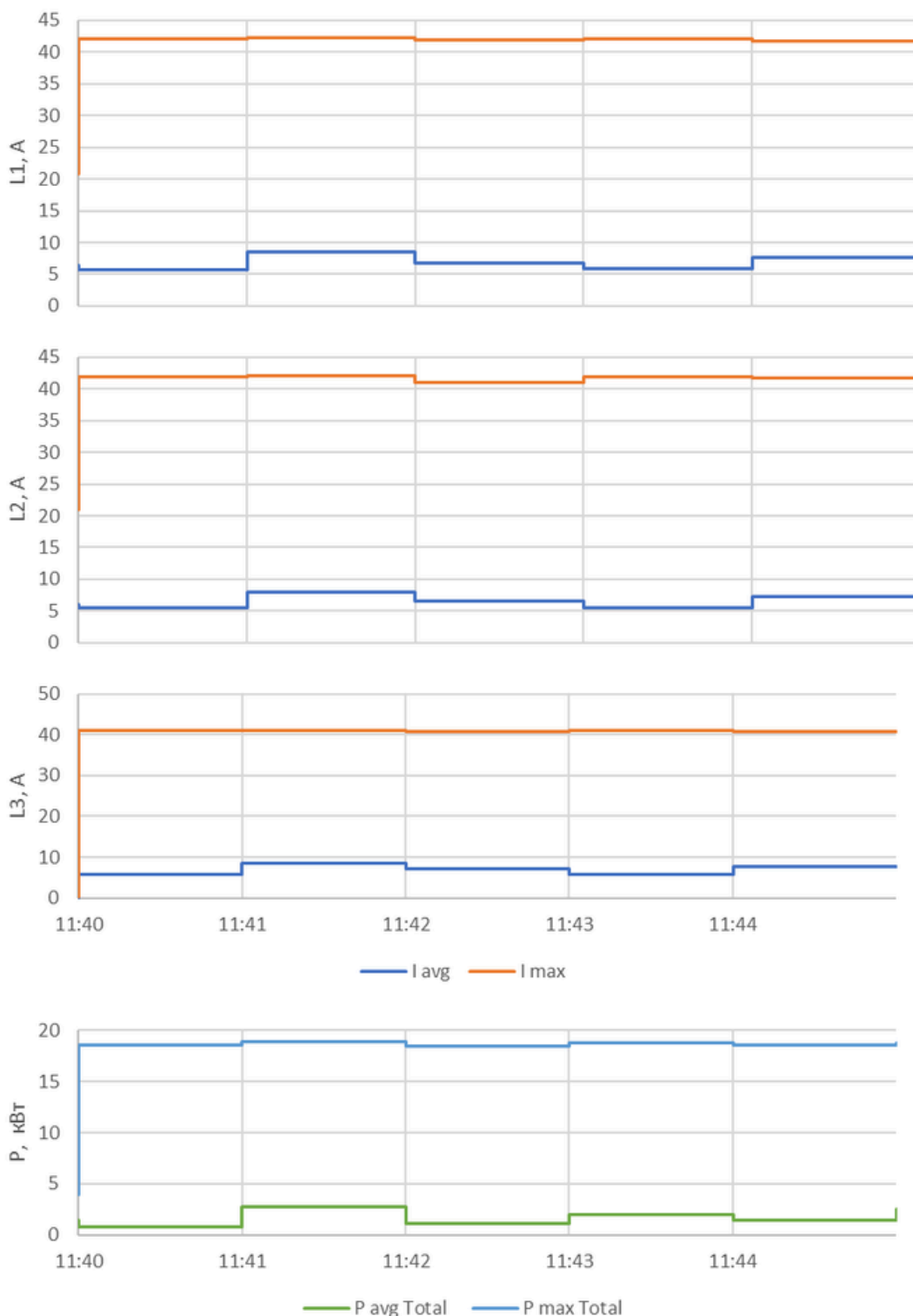
Рис. 2. Результати замірів пускових струмів під час роботи ліфта 400 кг 2-х швидкісний
