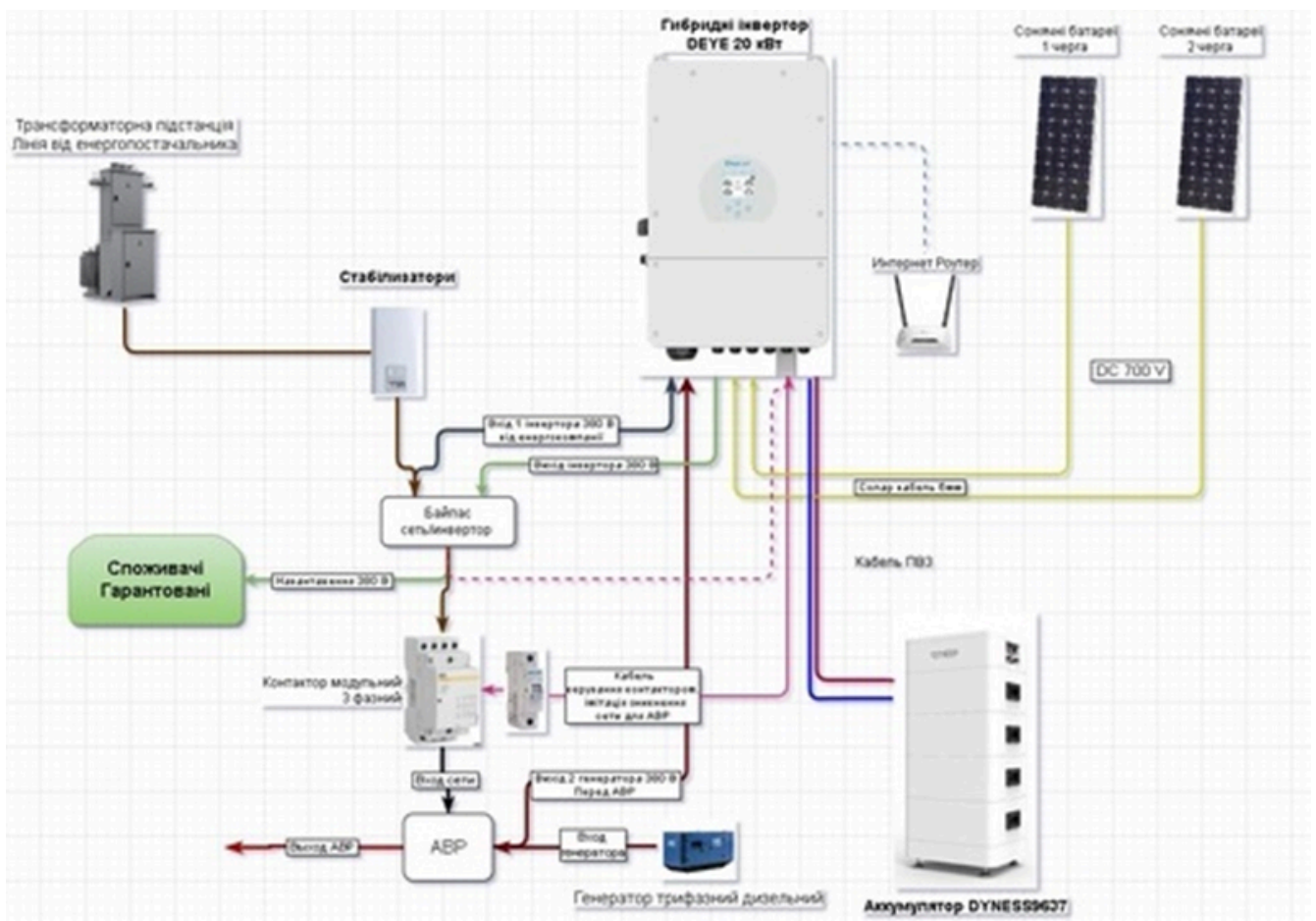
Рис. 2. Узагальнена схема включення гібридного інвертору в загальнобудинкову мережу
