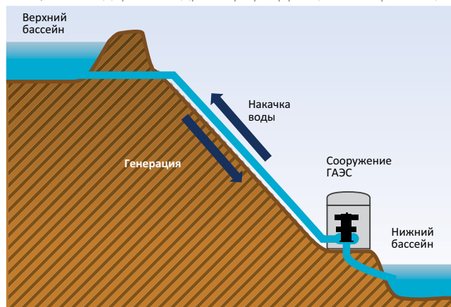
Рис. 7.10. Стандартная гидроаккумулирующая электростанция
