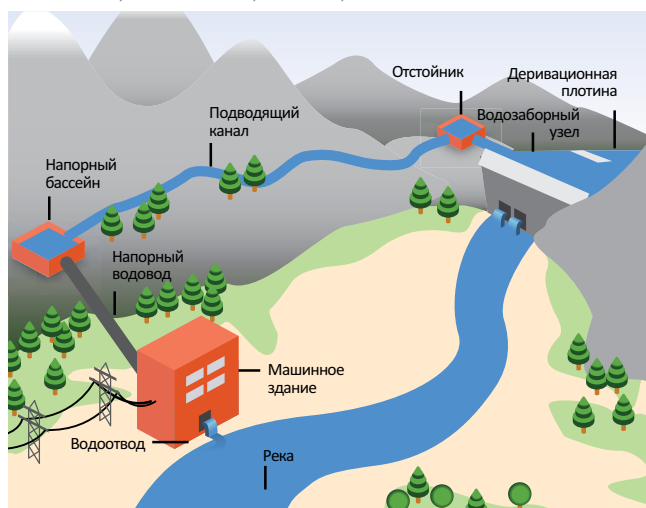
Рис. 7.8. Русловая гидроэлектростанция
