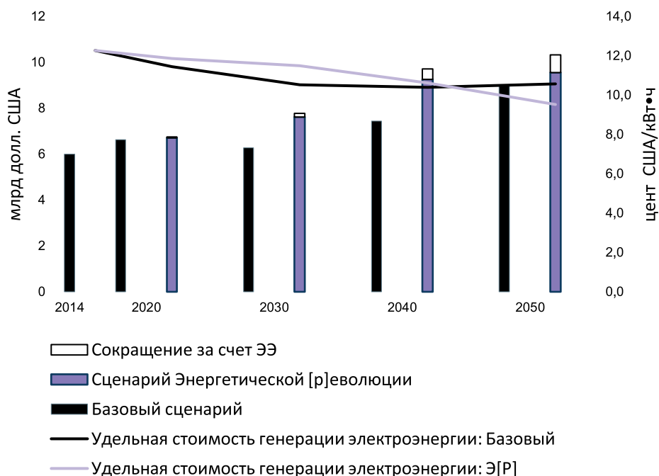
Рис. 6.6. Изменение общих затрат на электроснабжение и удельной стоимости производства электрической энергии
