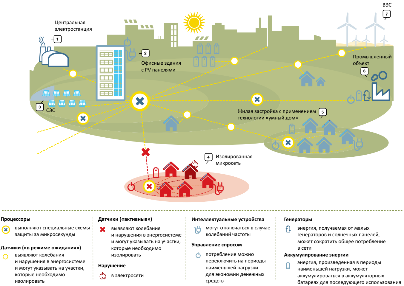
Рис. 2.4. Перспективы интеллектуальных электросетей в контексте Э[Р]
